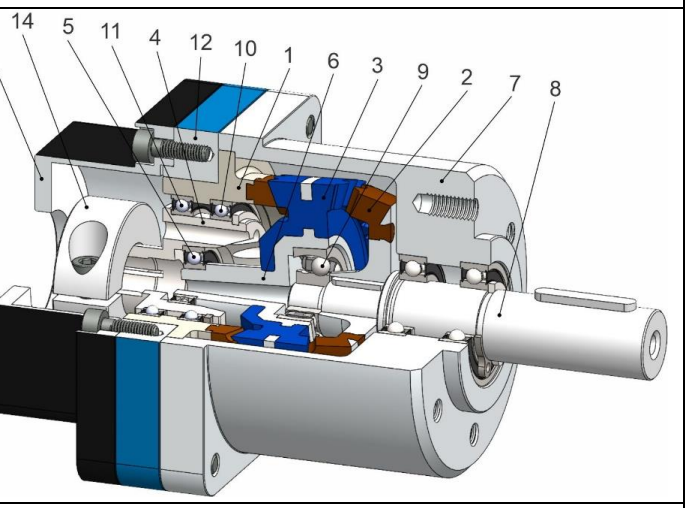
Transmisii precesionale cu coraportul dinților: Z_1 = Z_2 - 1, d_{(1-2)} = 22^\circ 30' și Z_4 = Z_3 - 1, d_{(3-4)} = 22^\circ 30'
