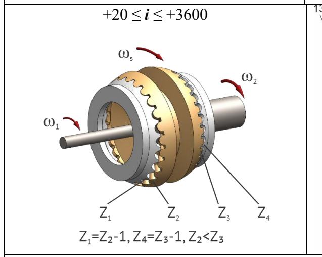
Transmisii precesionale cu coraportul dinților: Z_1 = Z_2 - 1, d_{(1-2)} = 22^\circ 30' și Z_4 = Z_3 - 1, d_{(3-4)} = 22^\circ 30'
