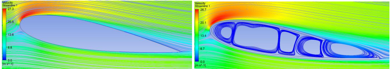
Liniile de curent și distribuția vitezelor în jurul palelor NACA 0018 închise și cu deschidere, unghiul de atac 10°.
