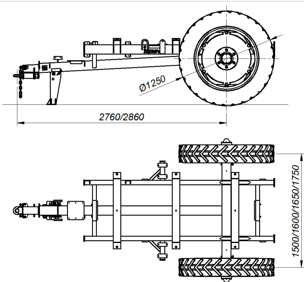
Fig.5.3.6. Noua construcție a șasiului pentru mașini cu capacitatea rezervorului 2 m 3
