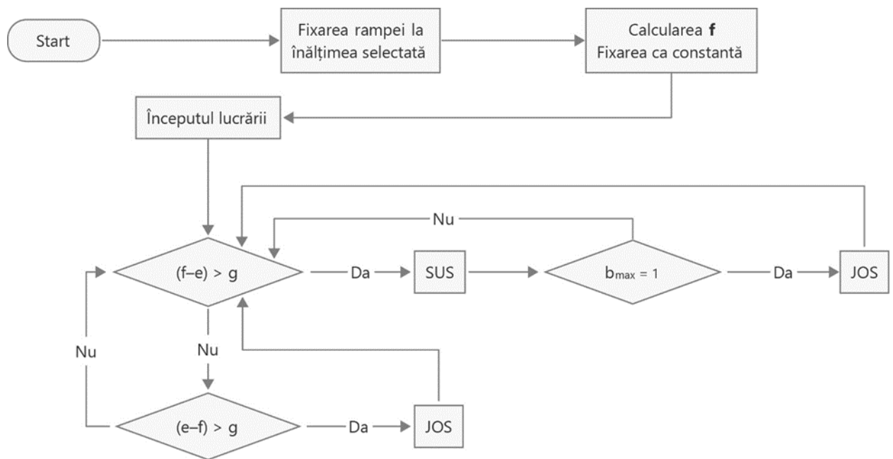
Fig. 5.5.2. Algoritm de funcționare a controlorului, unde f – distanța minimă până la sol (valoarea setată); g – histerezis (valoarea setată); b_{max} = 1 – punctul superior de ridicare a tijei.
