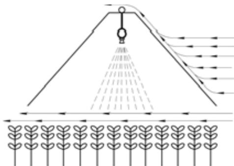
Fig.5.4.1 Protejarea jetului cu ajutorul apărătorii rigide
